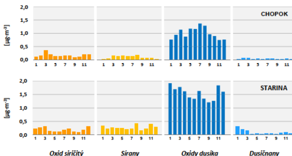
Obr. 3.2 Priemerné mesačné koncentrácie znečisťujúcich látok v ovzduší, rok 2022 (prepočítané na síru, resp. dusík).
