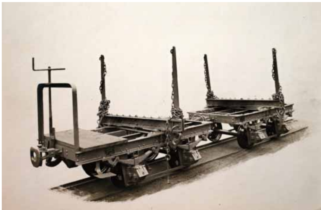
Oplenový vozeň, ktorým sa prevážalo drevo na lesnej železnici medzi Oščadnicou a dolinou Chmúra (Zdroj : Zbierkový fond Kysuckého múzea H 2405)
