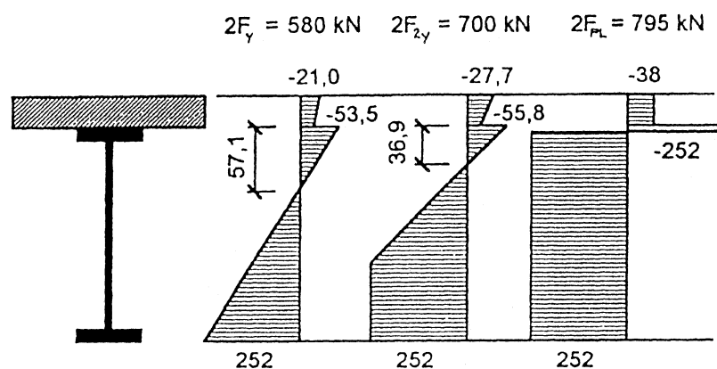
Obr. č. 3. Rozdelenie napätí a príslušné zaťaženie v pružnom, pružno-plastickom a plastickom štádiu pôsobenia trávov Fig. 3 Stress diagrams and ultimate load for elastic, elasto-plastic and plastic beam states
