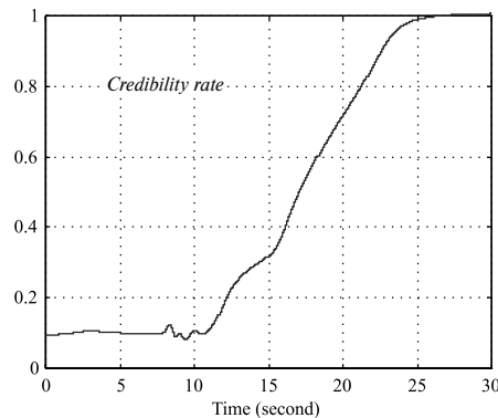
Obr. 4. Miera vierohodnosti údajov v1 pri chybe merania Fig. 4 Credibility rate of value v1 under measurement fault
