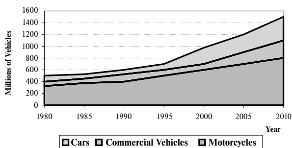
Obr. 1. Celkový trend vývoja motorových vozidiel [3] Fig. 1 Global trend in motor vehicles [3]
