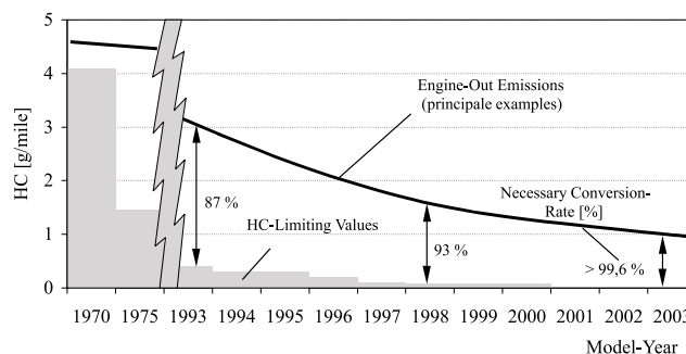
Obr. 7. Zníženie limitu pre emisie HC, požadovaná hladina zníženia HC a účinnosť katalyzátora podľa noriem US Fig. 7 Reduction in the HC emission limit, required reduction level in HC emission and catalyst efficiency for fulfilment of the US standards
