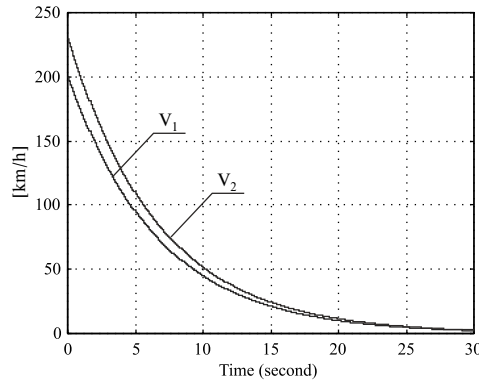
Obr. 3. Simulácia chyby merania rýchlosti Fig. 3 Simulation of velocity fault measurement
