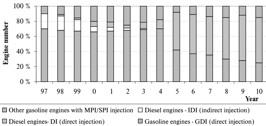
Obr. 4. Predpokladaný percentuálny podiel motorov na rôzne palivá pre automobily, ktoré sa budú vyrábať v EU v rokoch 1997-2010 [6] Fig. 4 Foreseen % share of engines with different fuel supply in cars to be manufactured in the EU in years 1997-2010 [6]
