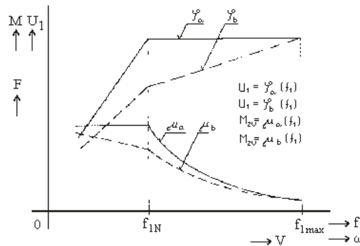
Obr. 4.1. Príklad priebehu vyšetrovaných medzných mechanickej charakteristik \mu_a a \mu_b pre rôzne priebehy riadenia statorového napätia \varphi_a a \varphi_b
