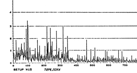
Obr. 7. Analýza prejazdu lokomotíva rýchlosť 96 km/h Fig. 7 Analysis of the locomotive passage, speed 96 km/h
