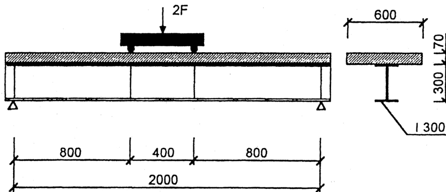
Obr. č. 2. Tvar a usporiadanie modelov spriahnutých trémov Fig. 2 Details of tested composite beams
